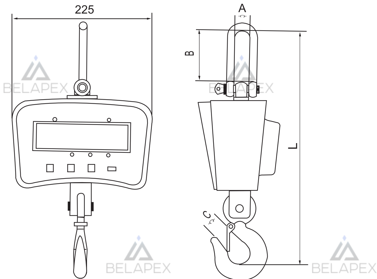
Рисунок 4.2 – Размеры весов
